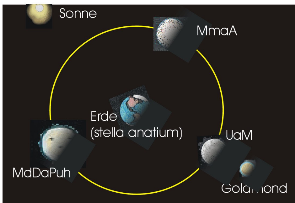
Abb. 22b: Schematische Darstellung der Abschattungen der Himmelskörper
